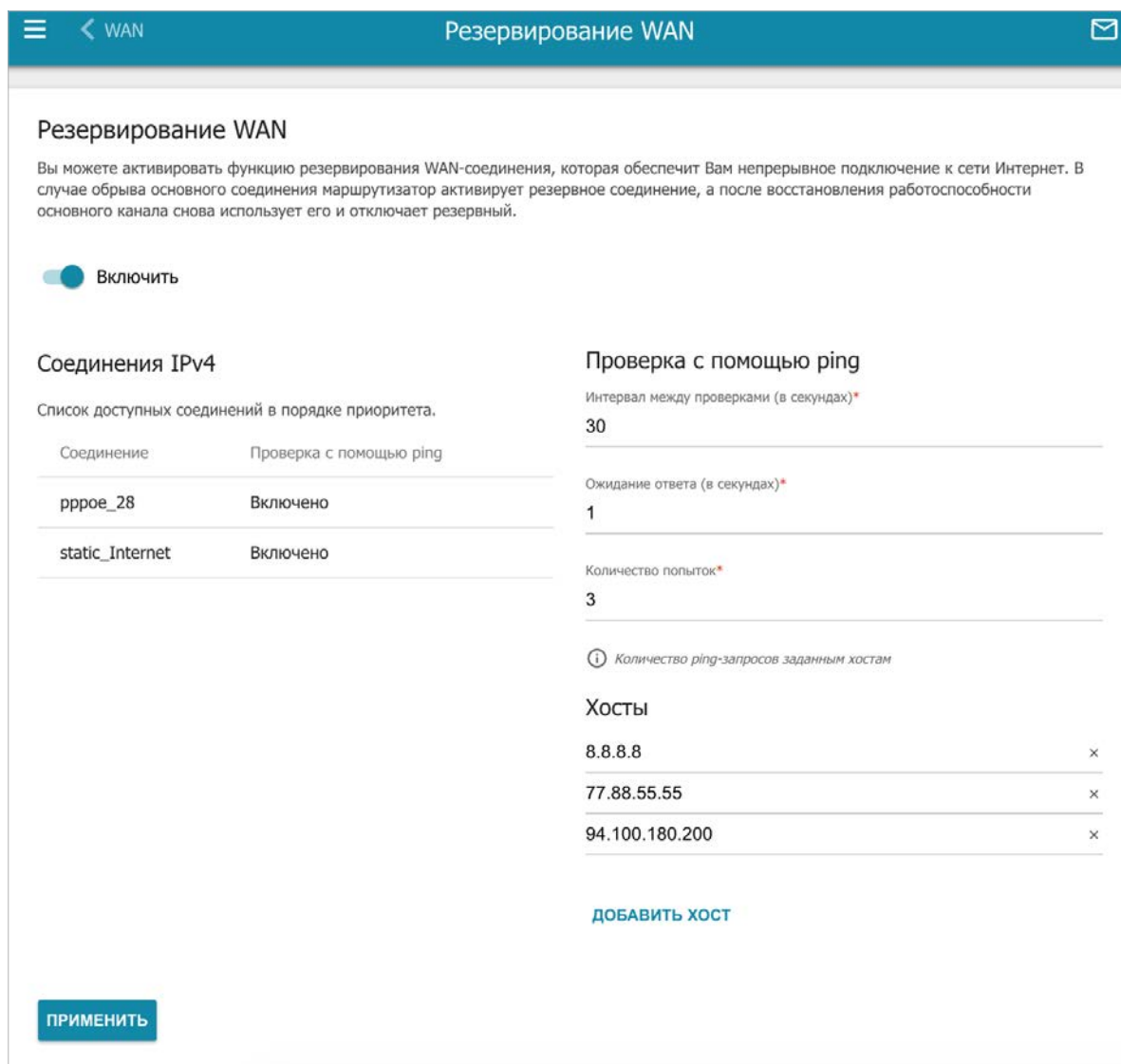
Рисунок 103. Страница Настройки / Резервирование WAN .
